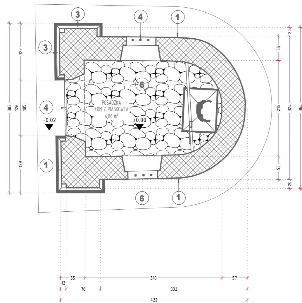
RZUT PRZYZIEMIA
